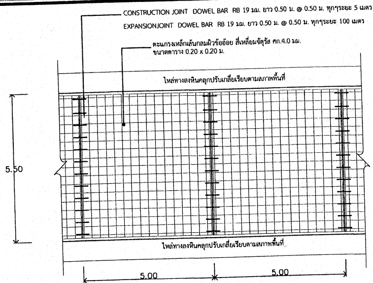
แปลนแสดงการเสริมเหล็กและรอยต่อถนน คสล.
