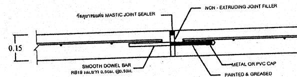
ขยายรอยต่อ EXPANSION JOINT
