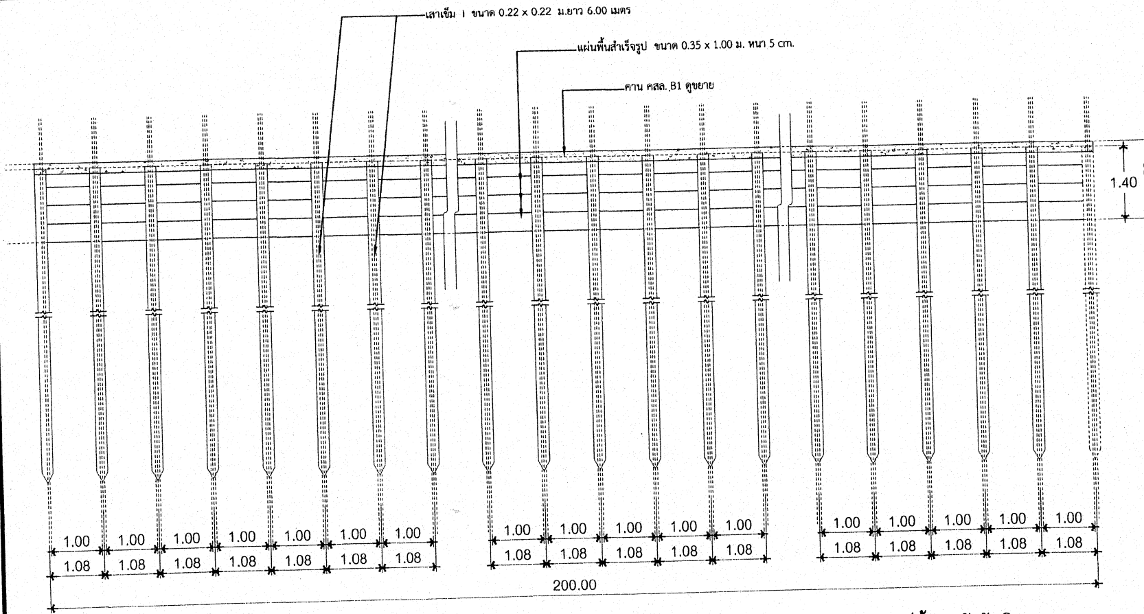
รูปด้านผนังกันดิน
