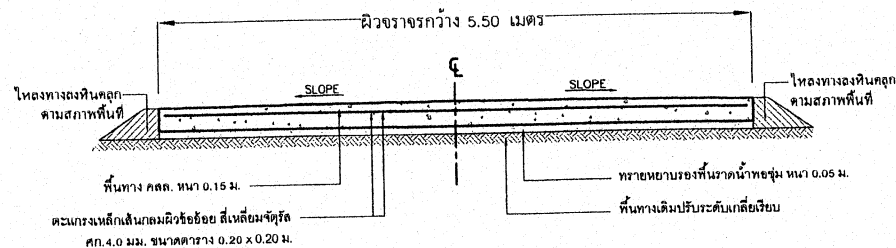
รูปตัดถนน คสล. A-A NOT TO SCALE
