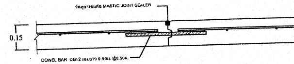
ขยายรอยต่อตามยาว LONGITUDINAL JOINT
