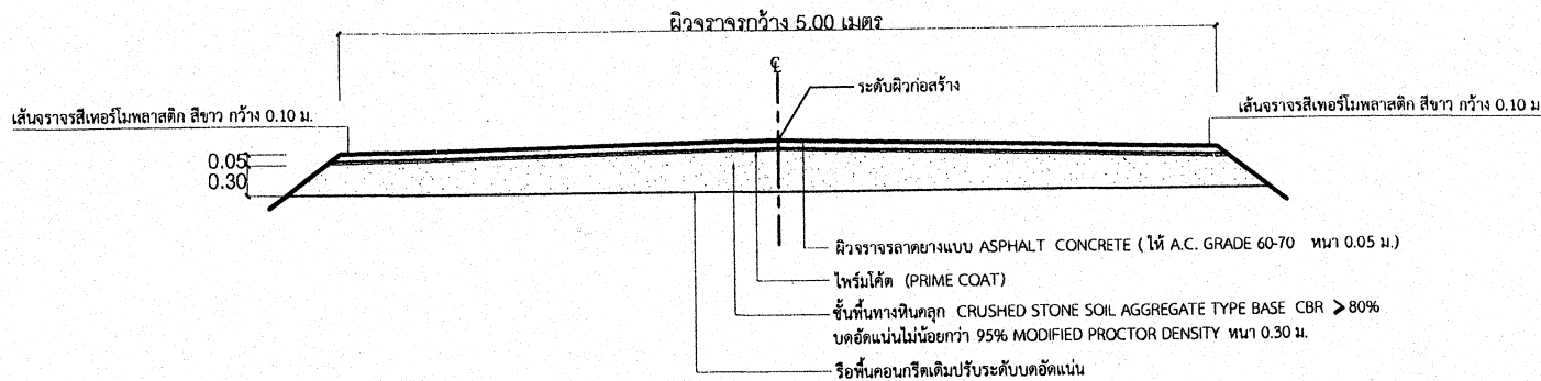
รูปตัด A - A ถนนแอสฟัลต์คอนกรีต
