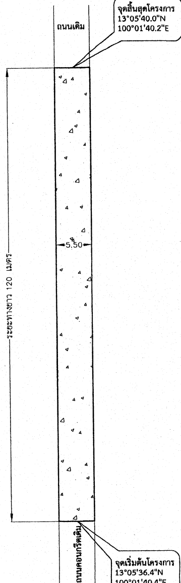
แปลนความยาว ถนน คสล. NOT TO SCALE
